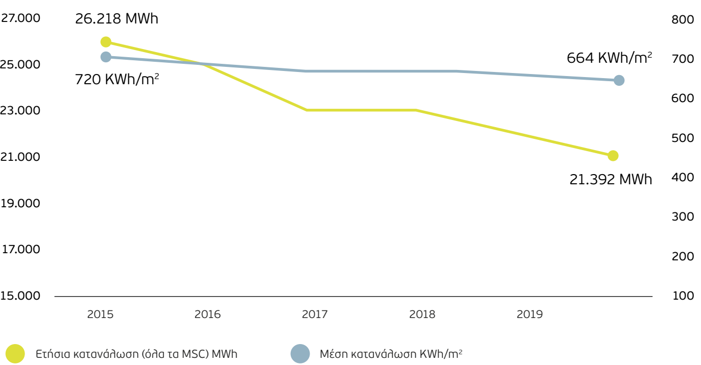
ΣΧΗΜΑ 3: Εξέλιξη κατανάλωσης ηλεκτρικής ενέργειας στα κτίρια και σχετικής κατανάλωσης (ανά τ.μ.) 2015-2020.
